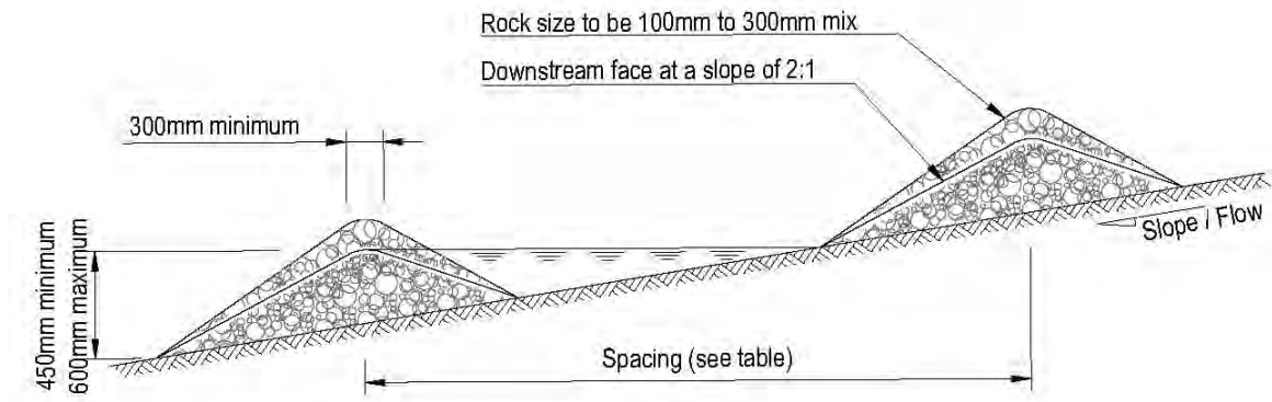
Elevation
